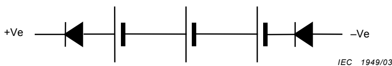
Figure E.2 – Mise en place de diodes de blocage pour répondre à E.4.3 (troisième exemple)
