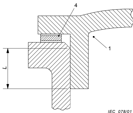
Figures 10 à 16 – Illustration des exigences relatives aux garnitures d'étanchéité
