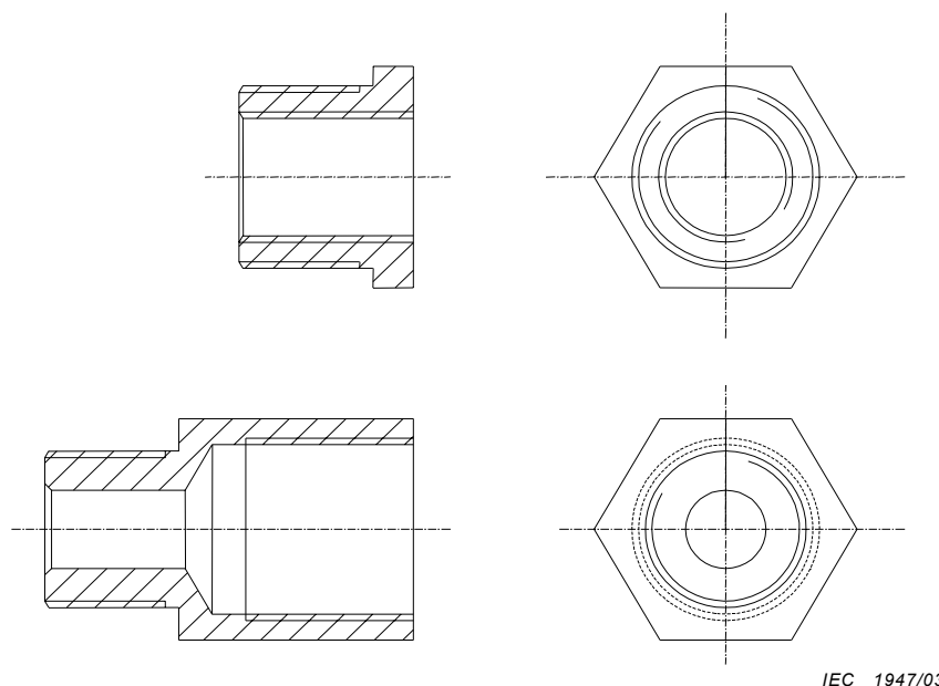
Figure C.2 – Exemples d'adaptateurs filetés Ex
