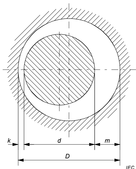
Figure 20 – Joints des traversées d’arbre de machines électriques tournantes
