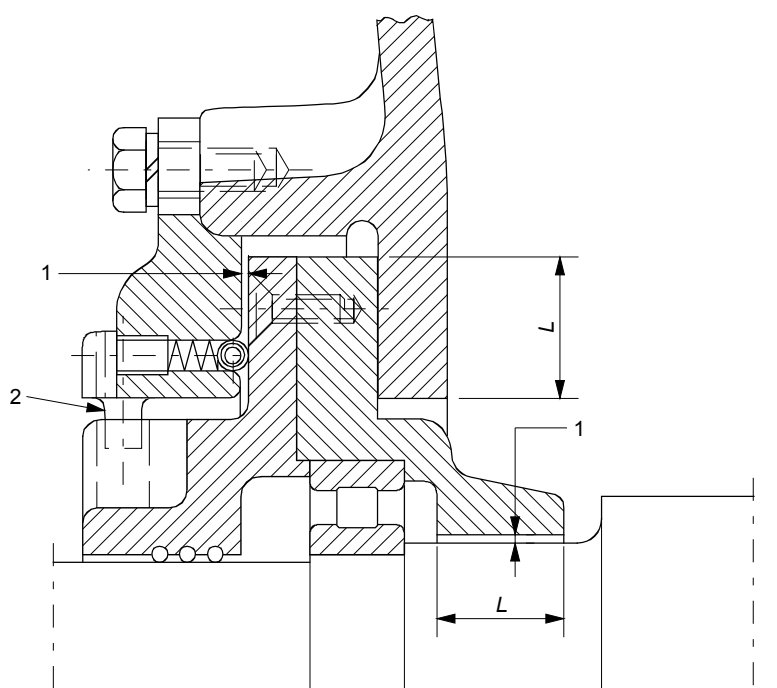
Figure 18 – Exemple de joint à labyrinthe pour arbre de machine électrique tournante
