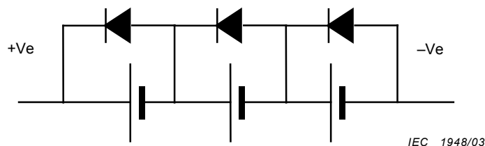
Figure E.1 – Montage de diodes pour trois éléments en série
