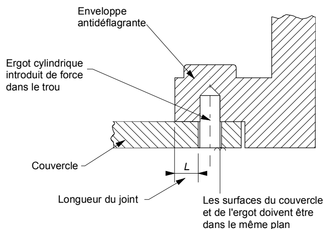
Figure 1 – Exemple de construction pour la vérification indirecte d'un joint plan antidéflagrant du Groupe I
