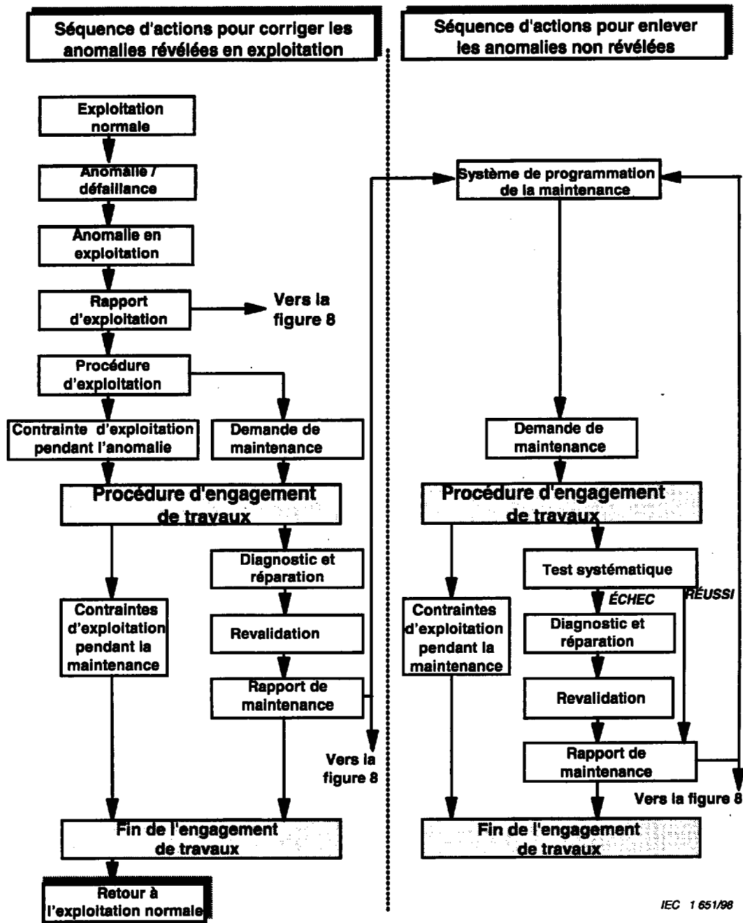
Figure 7 – Exemple de modèle d'activités d'exploitation et de maintenance
