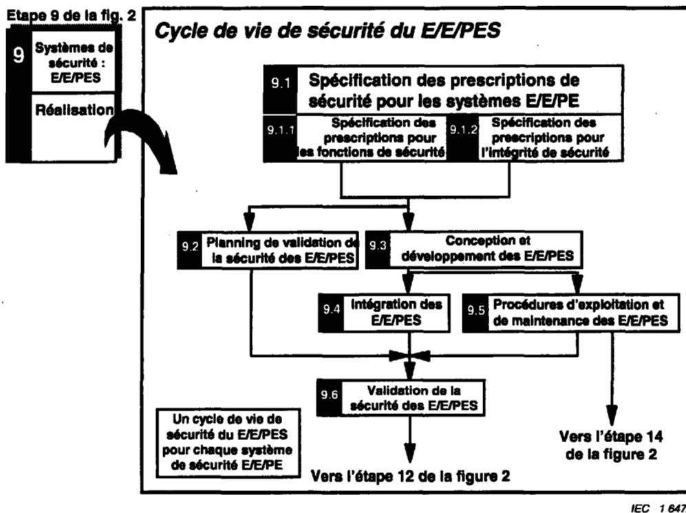
Figure 3 – Cycle de vie de sécurité du système E/E/PE (dans la phase de réalisation)
