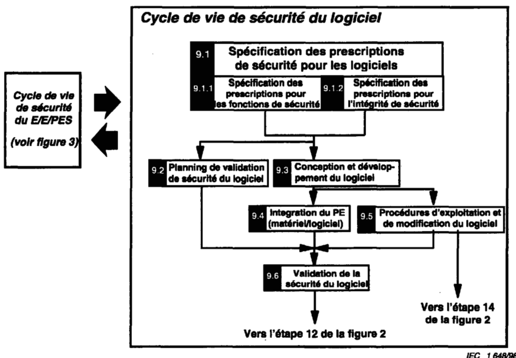
Figure 4 – Cycle de vie de sécurité du logiciel (dans la phase de réalisation)
