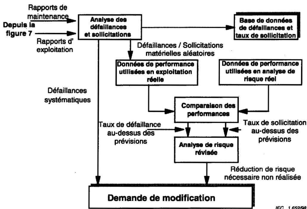
Figure 8 – Exemple de modèle de gestion de l'exploitation et de la maintenance
